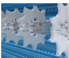
Pignone UltraClean per nastri modulari uni
